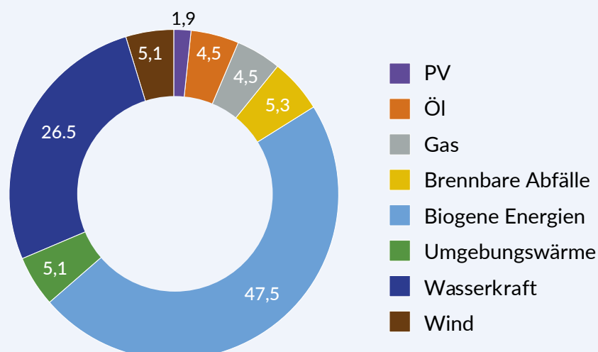
Brutto-Stromerzeugung in Österreich nach Erzeugungsquelle in Prozent (2021)
